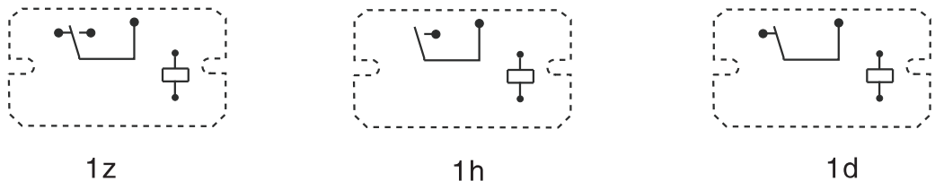
接线图
